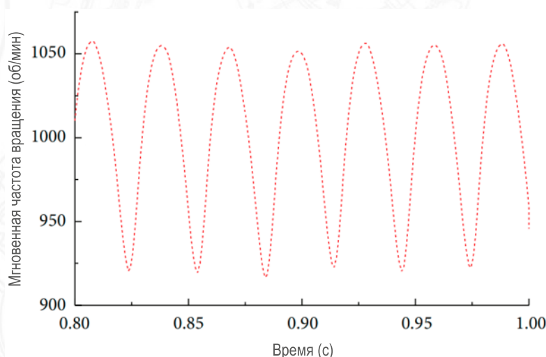
Амплитуда частоты вращения двигателя на холостом ходу (низкой) скорости.
