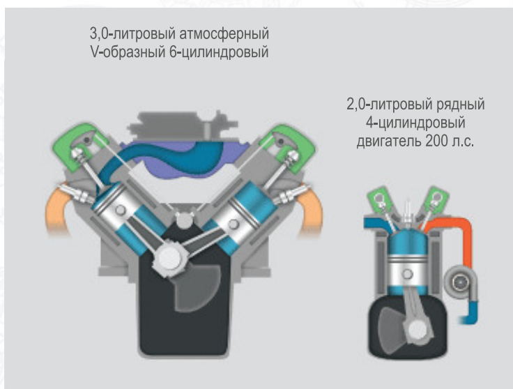
Уменьшение объема двигателя, компенсируемое наддувом с V-образного 6-цилиндрового двигателя до рядного 4-цилиндрового двигателя.
