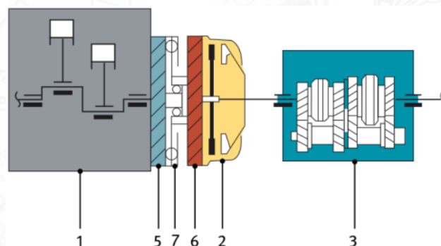
Принцип работы с двухмассовым маховиком (DMF)
