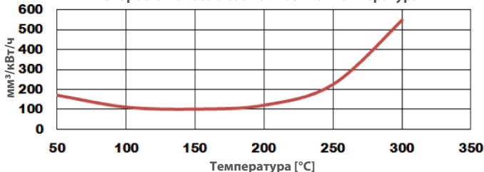
Скорость износа в зависимости от температуры
