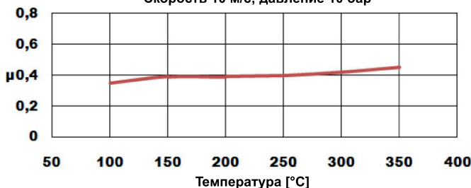
Коэффициент трения по сравнению с температурой Скорость 10 м/с; давление 10 бар
